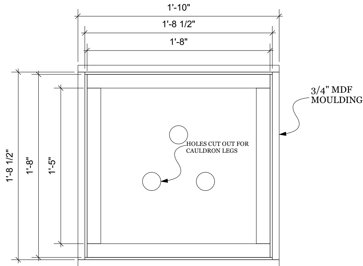
1 TOP VIEW Scale: 2" = 1'-0"
