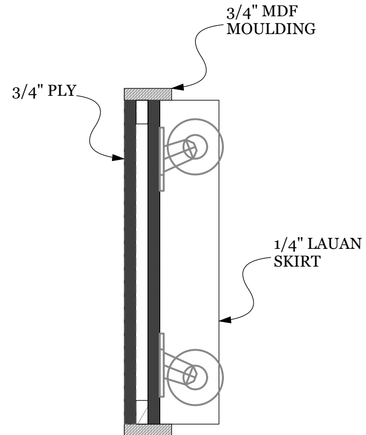
3 SECTION VIEW Scale: 2" = 1'-0"
